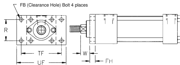
Mount Code F1 NFA MF1
