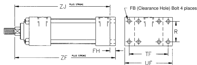
Mount Code F2 NFA MF2
